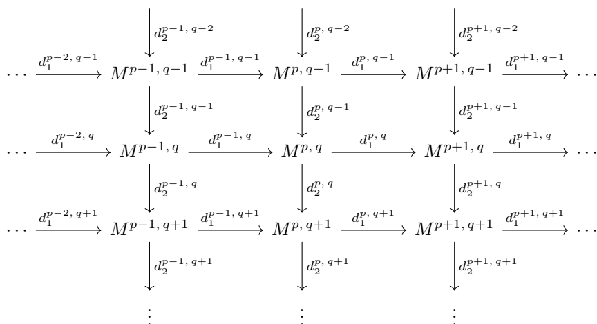
図 4.3: 二重複体
